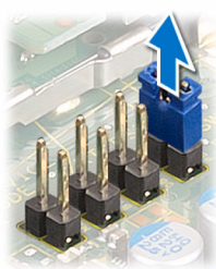
1 siltauskytkin
